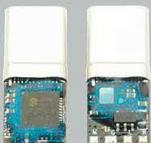
TYPE-C数字音频 HRW-TPV89 DAC:SPV6040 / 32Bit-384KHZ 带 AI-ENC 降噪
