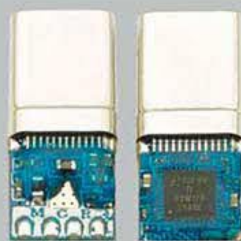
TYPE-C数字音频 HRW-TPV87 DAC:KT02F20 / 32Bit-192KHZ
