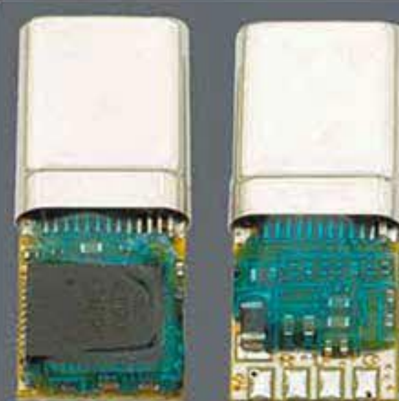
TYPE-C数字音频 HRW-TPV57 DAC:ALC5686 / 32Bit-384KHZ
