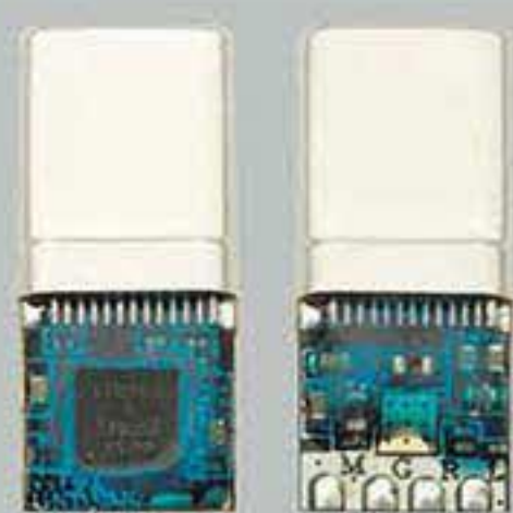
TYPE-C数字音频 HRW-TPV63 DAC:KT02H20 / 32Bit-384KHZ
