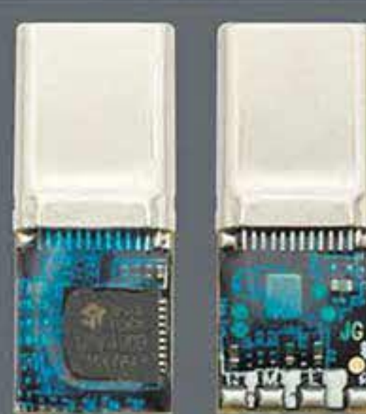
TYPE-C数字音频 HRW-TPV69 DAC:SPV4040 / 32Bit-3号4KH7 支持DSD256KHZ硬解
