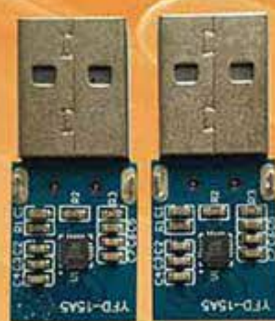
USB 音频蓝牙芯片
