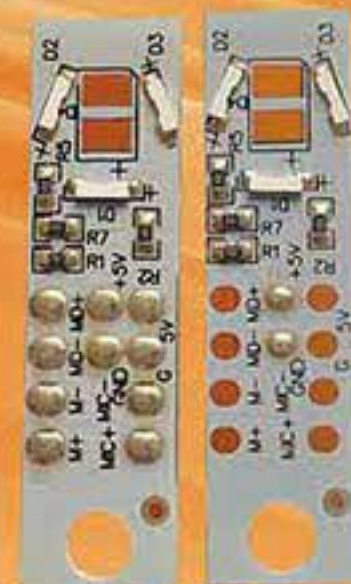
头戴耳机灯板
