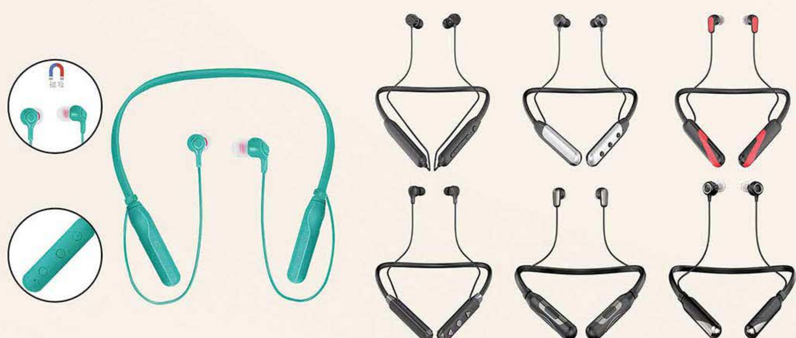
FY-45#3(单耳) 专利号: 202330213725.9 电池: 450845-150毫安 喇叭规格: 10厘 Type-C/数显 FY-45#1(单耳) 专利号: 202330213725.9 电池: 450845-150毫安 喇叭规格: 10厘 Type-C/数显 FY-47(单耳) 电池规格: 601045-250毫安 喇叭规格: 10厘 Micyo FY57# 专利号: 202430219446.8
